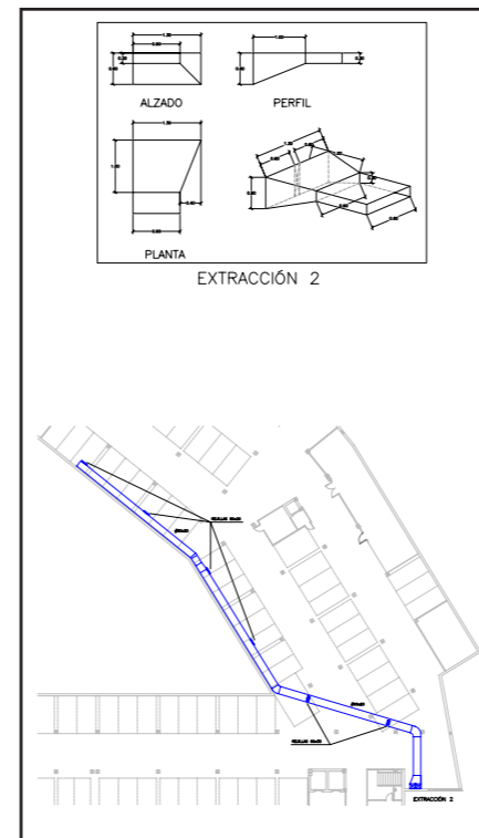
VENTILACIÓN PÁRKING
