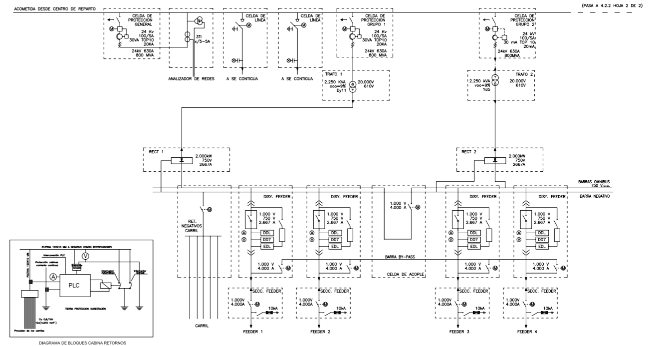
Esquema Unifilar Subestaciones 2 y 3
